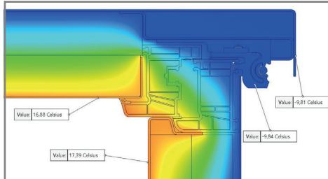
Şekil 1. Kompozit Menteşe
