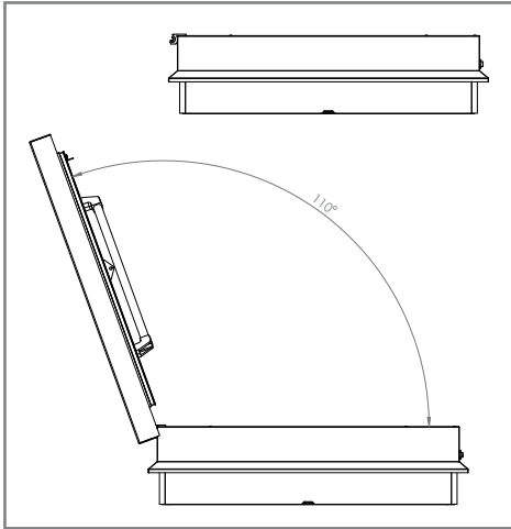
Şekil 4. 110° açılma açısı
